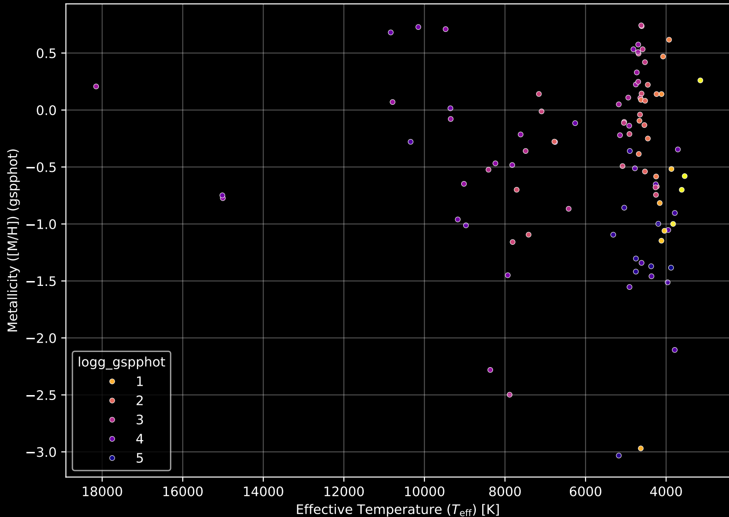
APOGEE DR17 Field: [005+00] Stellar Population Parameters (n= 96)
